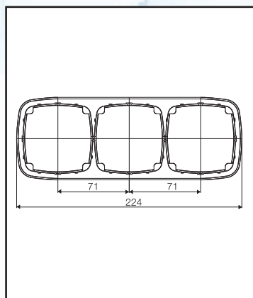
Trojrámček MODUL 4 FA 127 29
