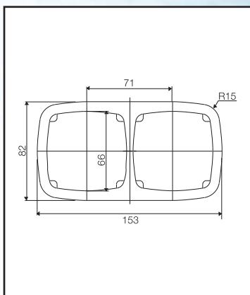
Dvojrámček MODUL 4 FA 127 28
