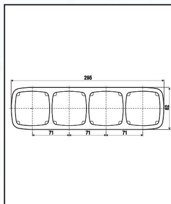
Štvorámček MODUL 4 FA 127 36
